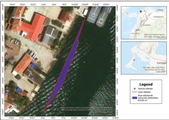
Imagen 5. Imagen solicitud de obras de BNL01 – área extracción de sedimentos.
