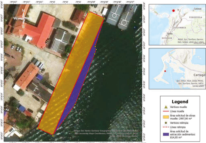
Imagen 16. Área de intervención de la solicitud de las obras en la Base Naval No. 1 ARC "Bolívar".
