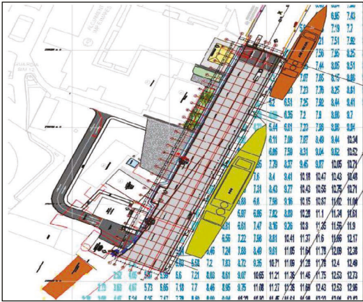
Imagen 6. Planos proyecto ampliación muelle embarcaciones mayores BN01.
