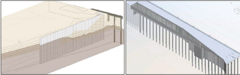
Imagen 8. Ubicación tablestacado tipo Larssen 600.
