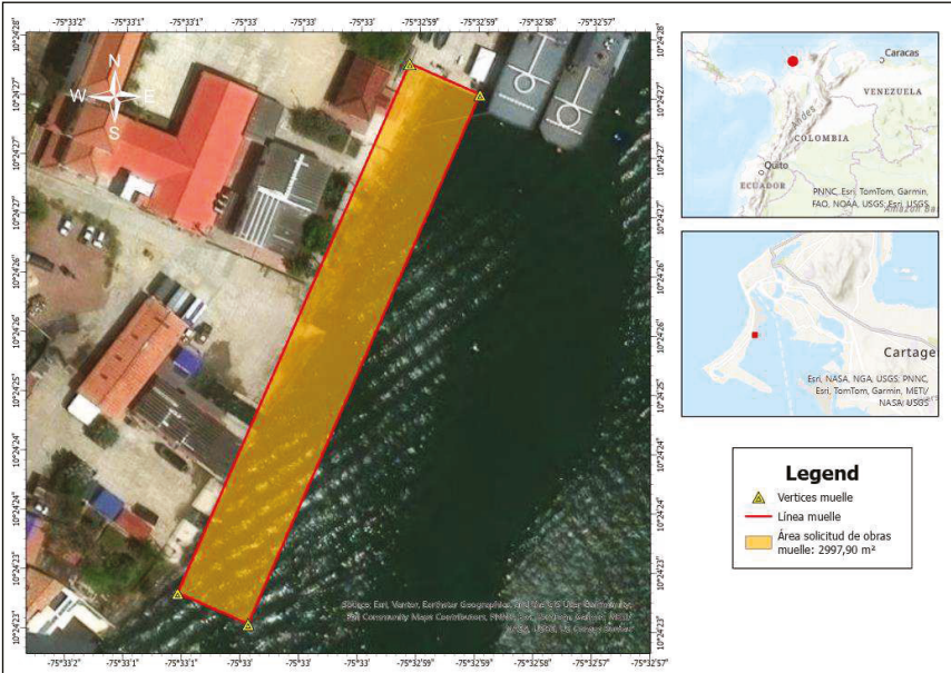
Imagen 14. Imagen solicitud de obras de BNL01 – área ampliación de muelle de embarcaciones mayores.
