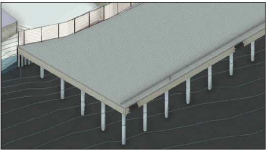
Imagen 7. Contención, soportes estructurales y cimentación del muelle. Fuente: Anexo Proceso Constructivo obras BNLI.
